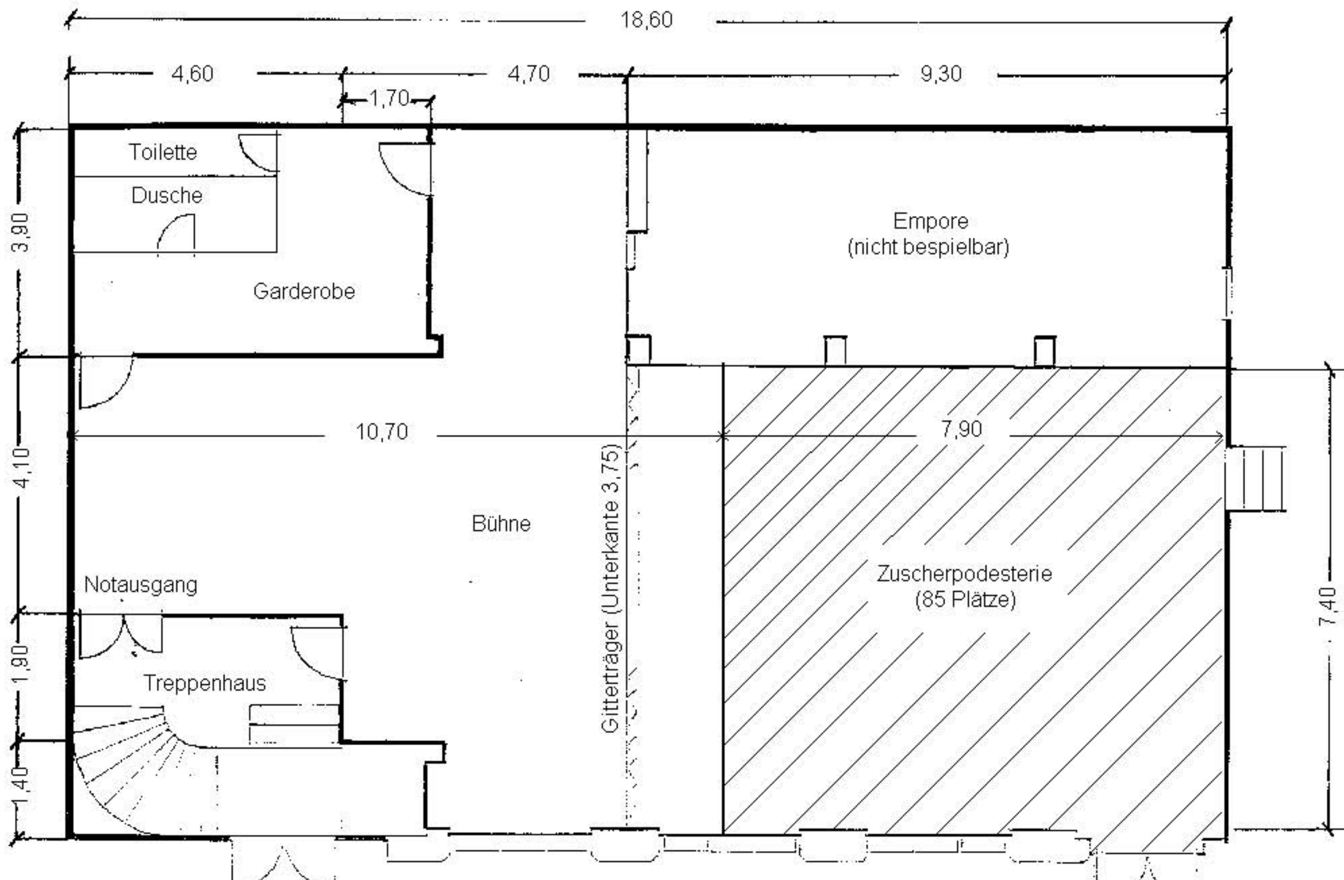
Theaterhaus Frankfurt Saal/Plan (alle Angaben in Meter)
